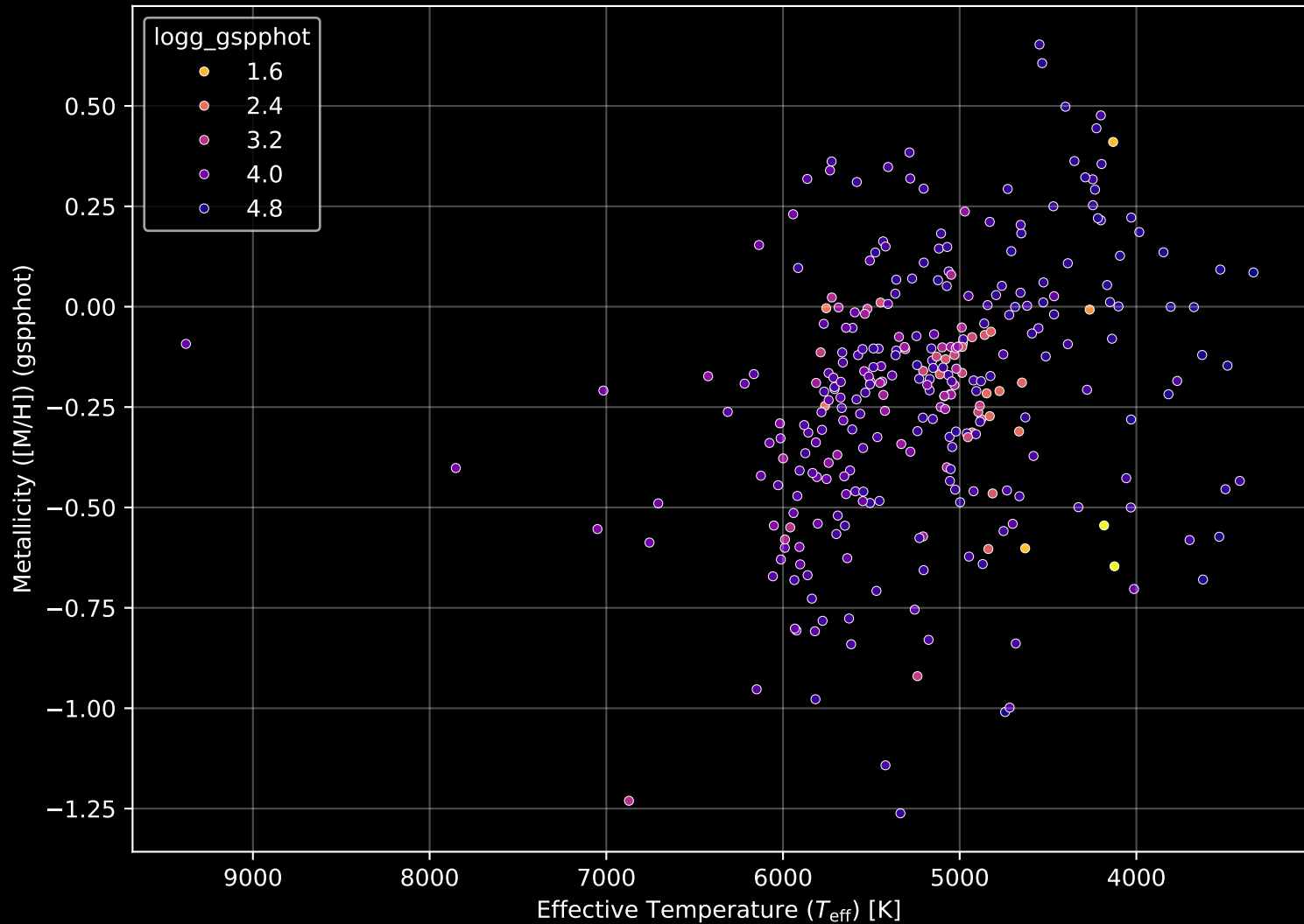
APOGEE DR17 Field: [220+55_btx] Stellar Population Parameters (n= 303)
